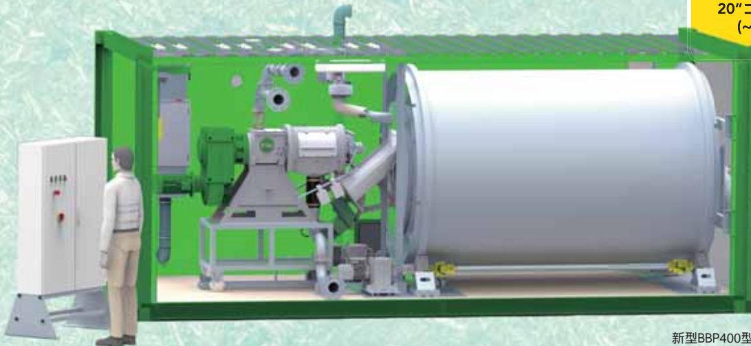
新型BBP400型
