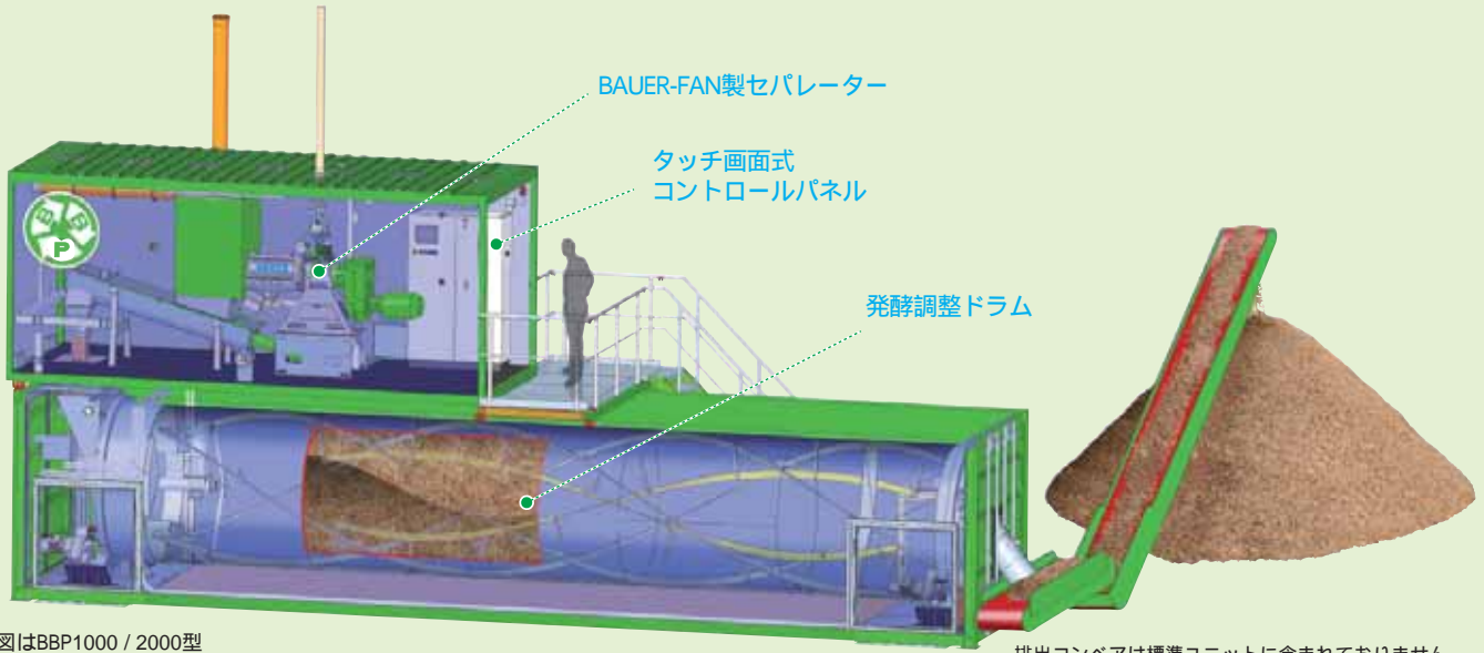
図はBBP1000 / 2000型
